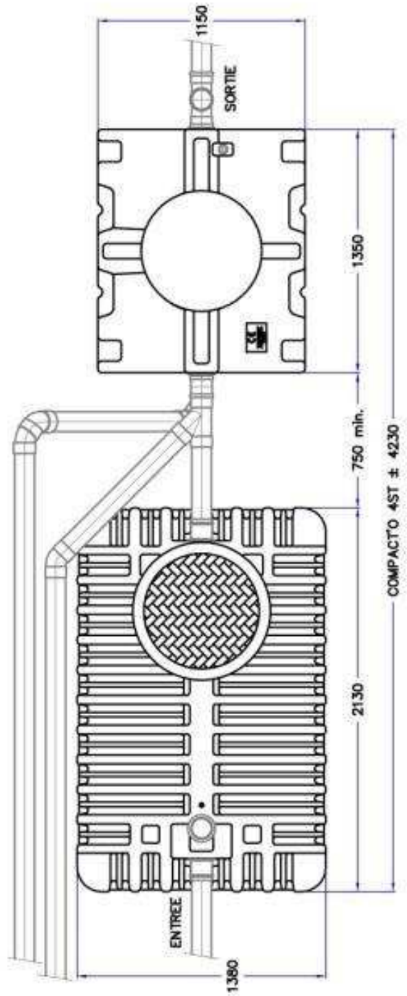
Fosse toutes eaux 3000 L
